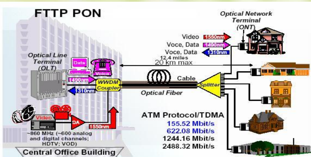
光纖到家 被動光纖網路架構圖
